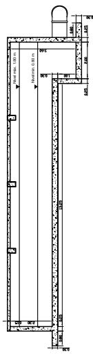
SECCIÓN D - D ESC. 1:100
