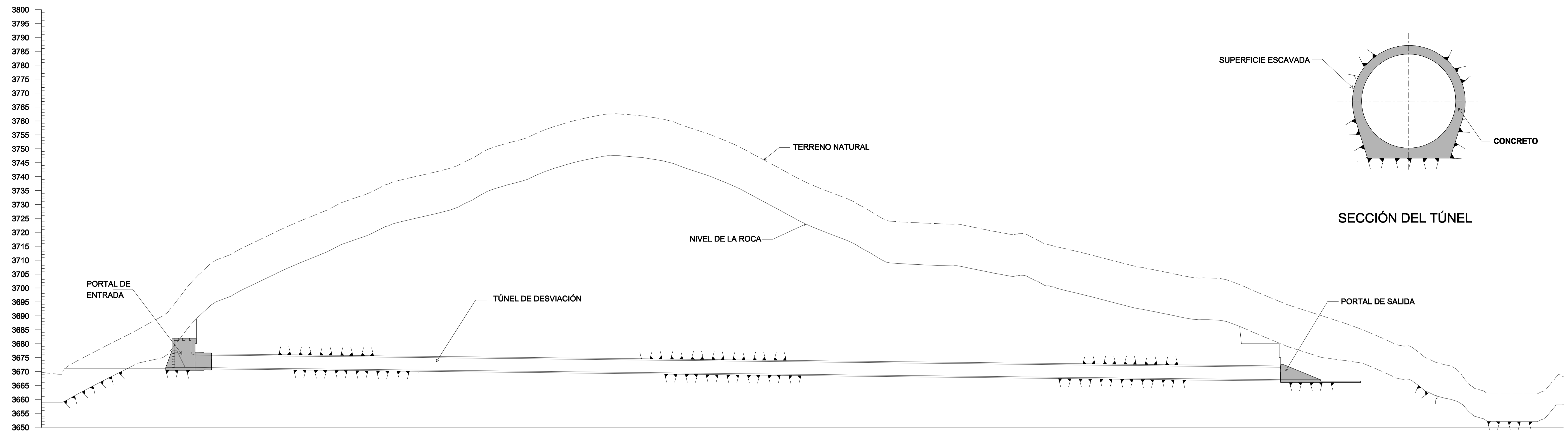
SECCIÓN C 1:750 TÚNEL DE DESVIACIÓN
