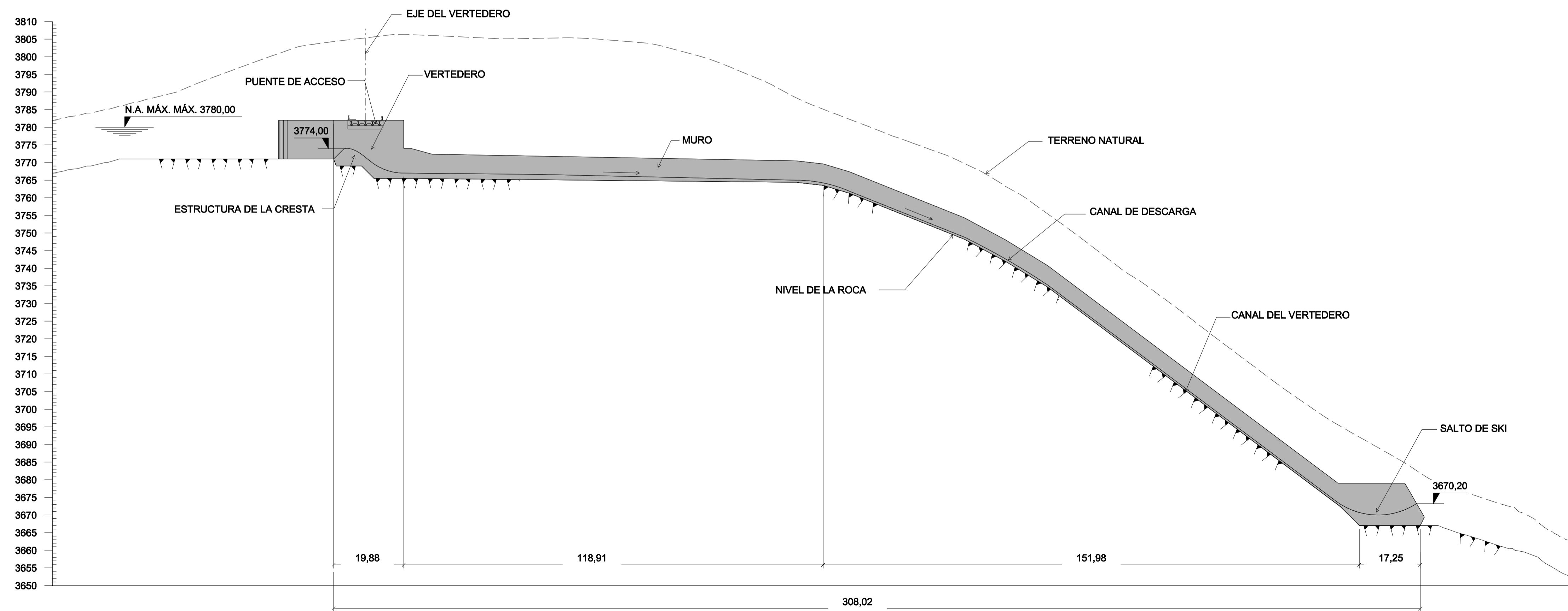
SECCIÓN D 1:750 VERTEDERO
