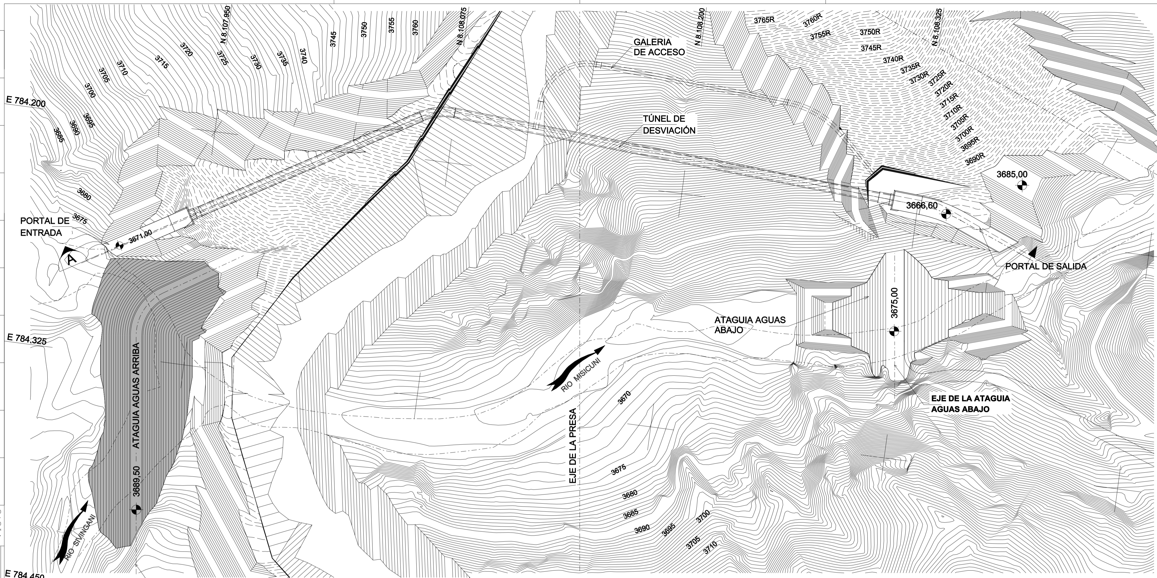
PLANTA 1:1000
