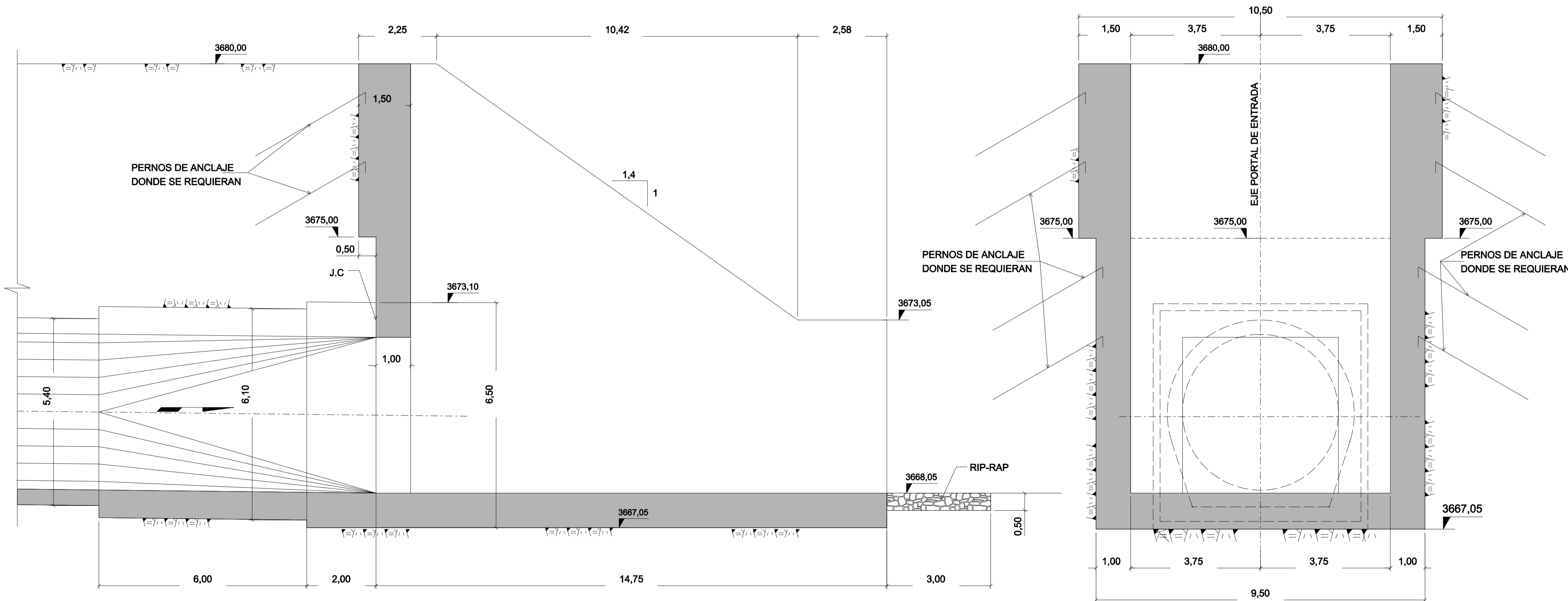
SECCIÓN A 1:75
