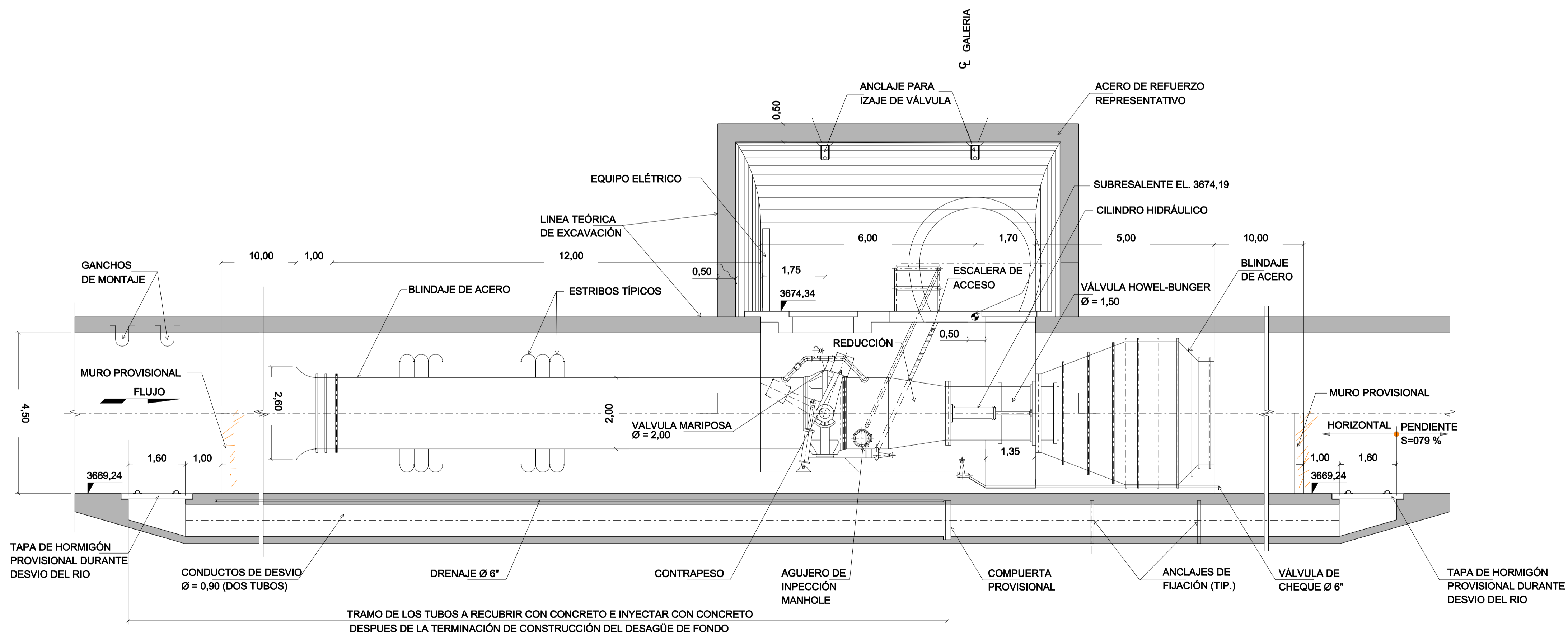
SECCIÓN A 1:75
